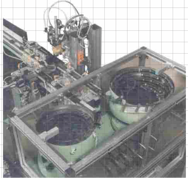
Separate Sortierungen und Zuführungen...
