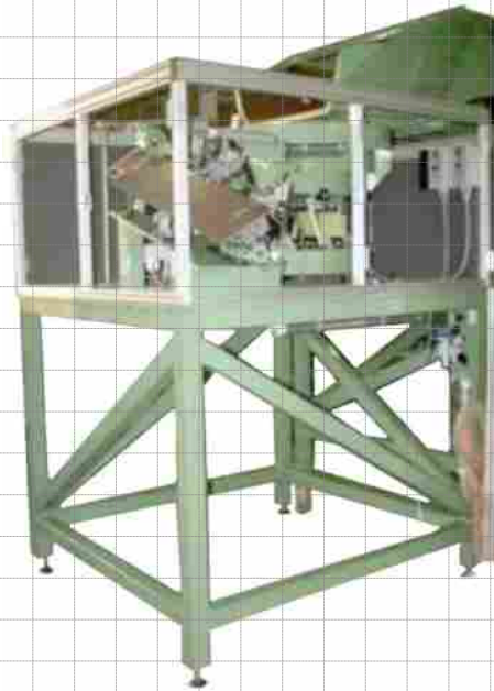
Sortierung und Zuführung der Schraubenrohlinge
