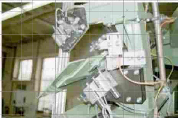
Zuführung und vereinzelte Bereitstellung zur Gewinderollmaschine
